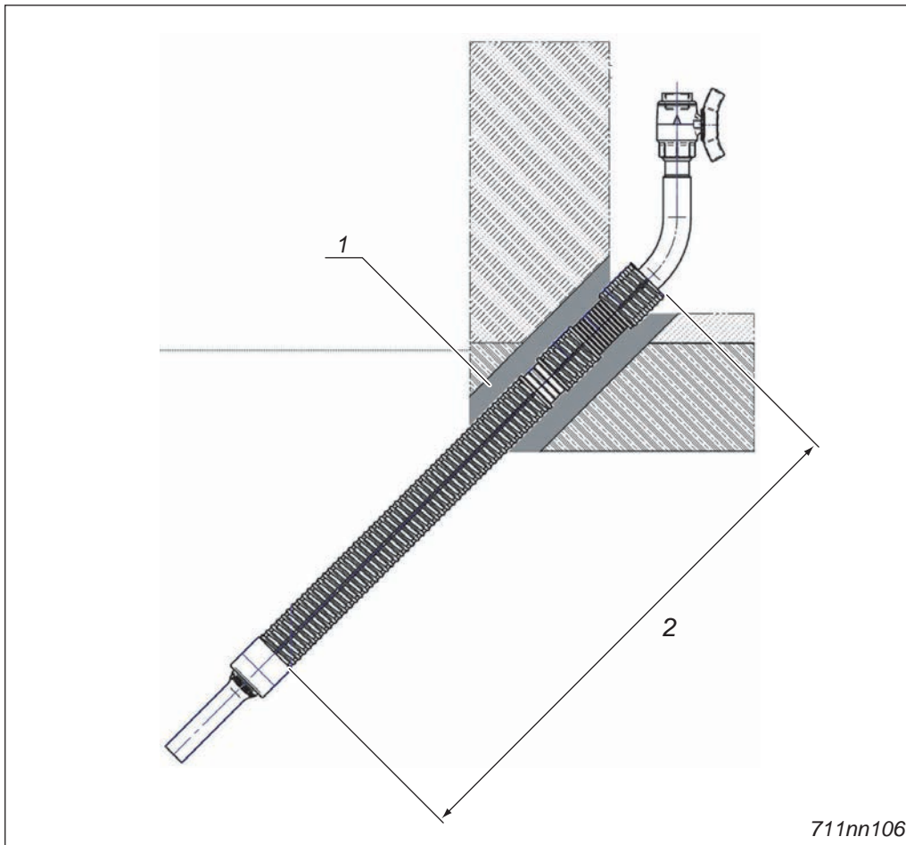
Fig. 4-6 DUO-FLEX 45°
