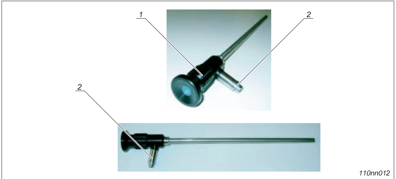
Fig. 3-3 Boroskop
